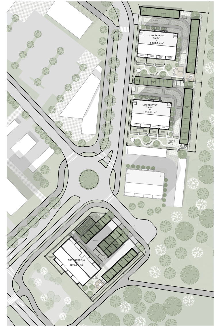
Asemapiirros 1:1500
