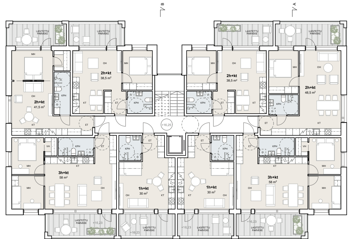
Pohjapiirros 2.-7. kerros 1:200
