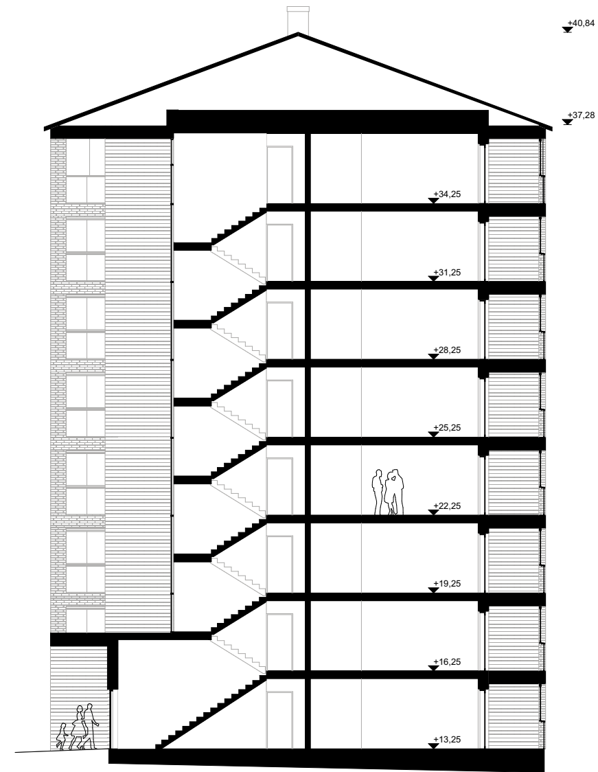
Leikkaus B-B 1:200
