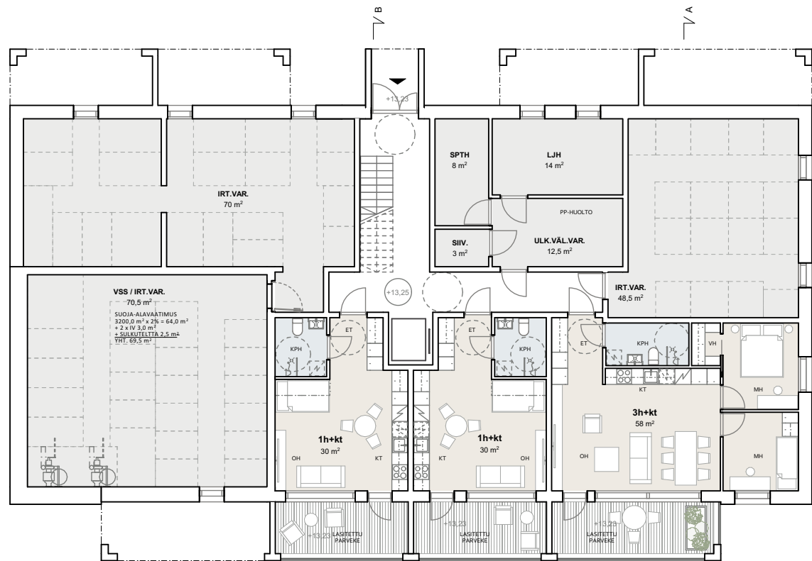
Pohjapiirros 1. kerros 1:200
