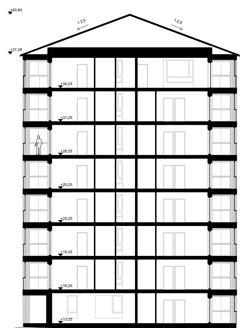
Leikkaus A-A 1:200
